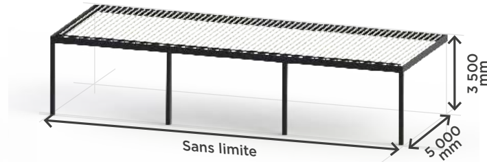
PergoToit Carport
