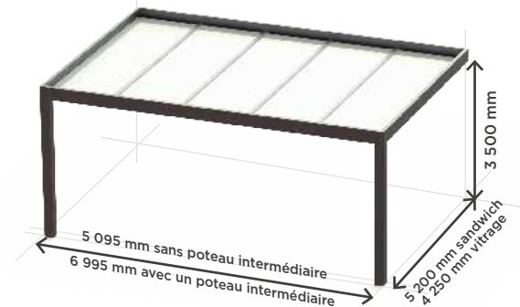
PergoToit Carport
