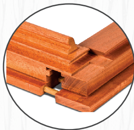
Assemblage des dormants et ouvrants en contre-profil et tourillons collés.
