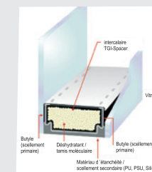
Coupe de l'intercalaire Warm Edge
