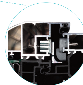
Conçu pour conserver et régler la compression sur la hauteur de l'ouvrant
