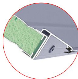
Couvre joint équipé d'un joint d'étanchéité
