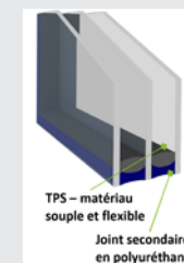
Coupe de l'intercalaire TPS
