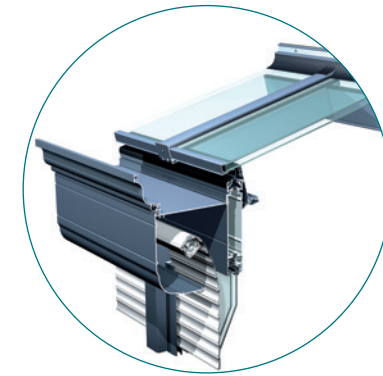
Intégration de coffre à volet roulant
