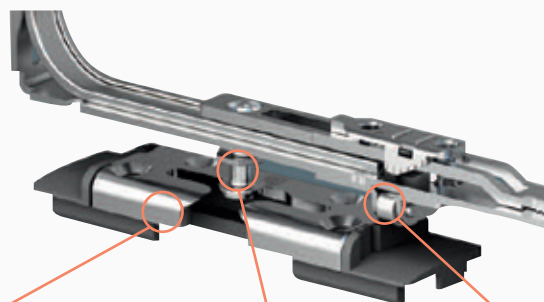
Gâche de sécurité en acier avec rampe inclinée
