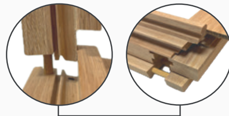
Assemblage des dormants et ouvrants en contre-profil et tourillons collés.
