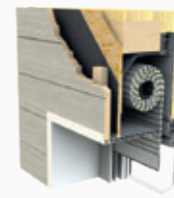
Demi-linteau ossature bois
