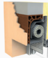
Demi-linteau maçonnerie traditionnelle
